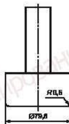
Рисунок 3 — Цилиндрический индентор
